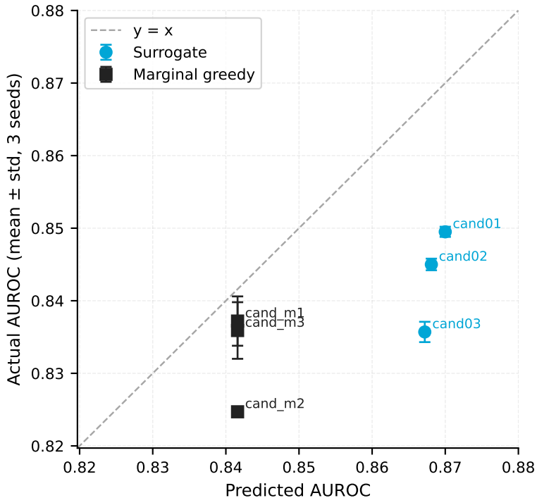
Predicted vs actual AUROC — Ch8 candidates
