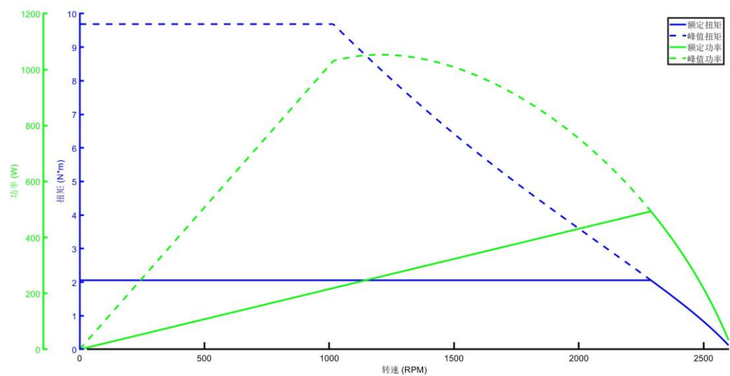
SEAF90A16NG01 关节电机外特性曲线
