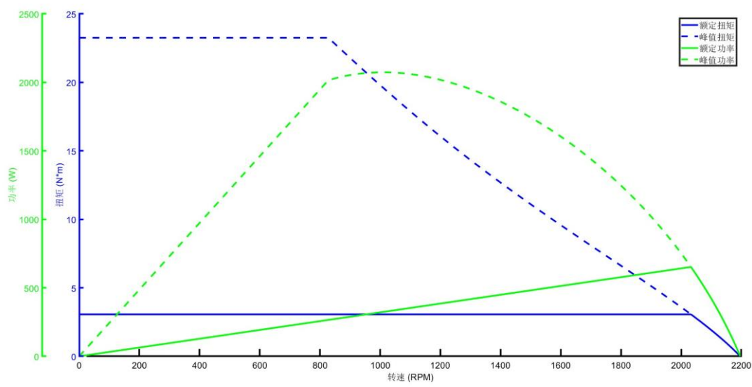
SETZ120CI-1JD 关节电机外特性曲线
