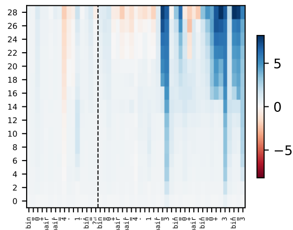
margin log p(true) - log p(lure)
