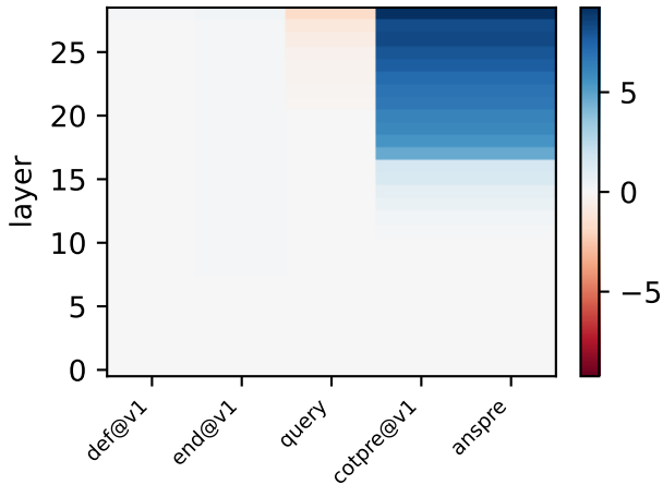
llama32-3b cot: \log p(\text{true}) - \log p(\text{lure})
