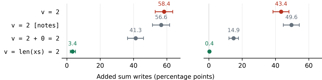
OLMo-2-7B-I
