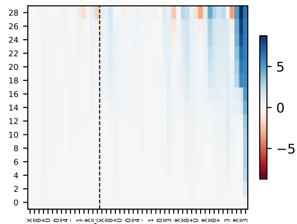
margin log p(true) - log p(lure)
