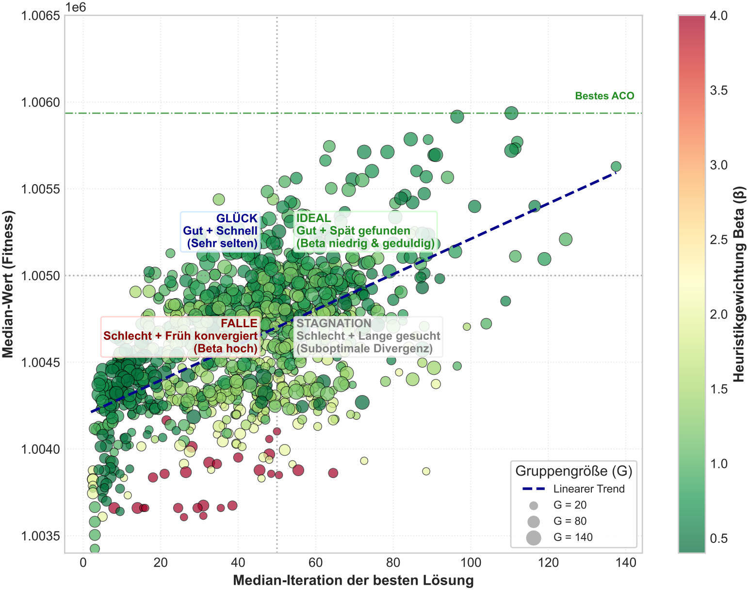
Konvergenzverhalten: Lösungsqualität vs. Suchdauer (Farbe repräsentiert Beta | Punktgröße repräsentiert Gruppengröße)
