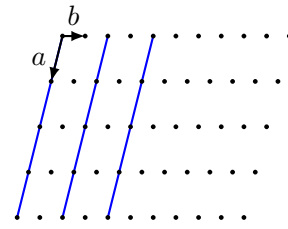
(f) 010
