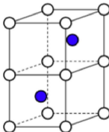
砷化镍（白：镍；蓝：砷）
