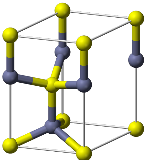
硫化锌（六方）
