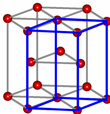
金属镁
