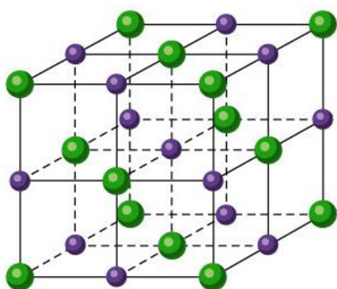
氯化钠
