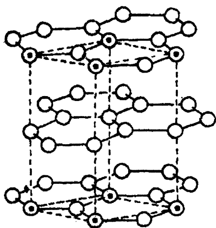
石墨
