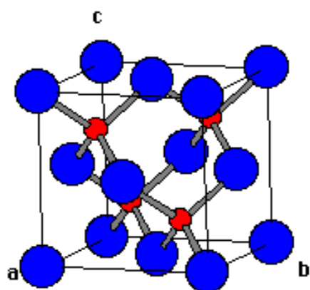
硫化锌（立方）
