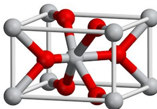
金红石
