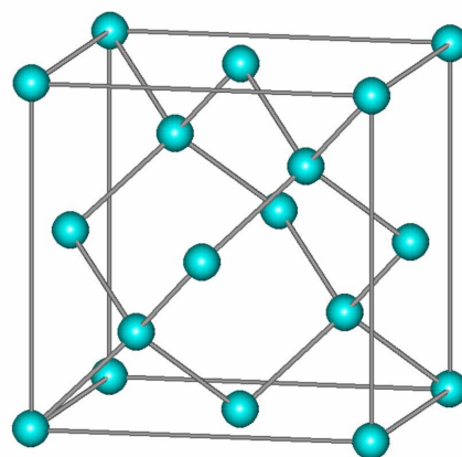
金刚石
