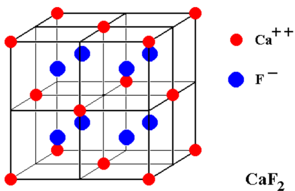
氟化钙
