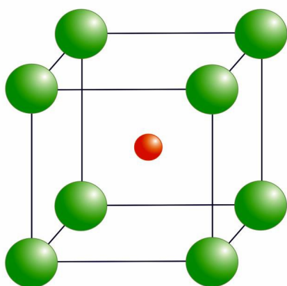
氯化铯
