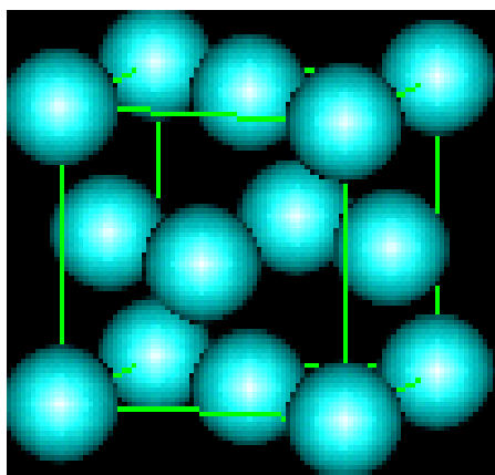
金属铜
