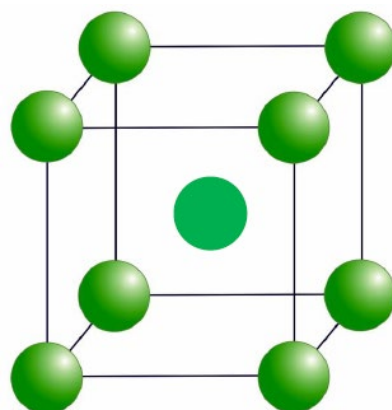
金属钠
