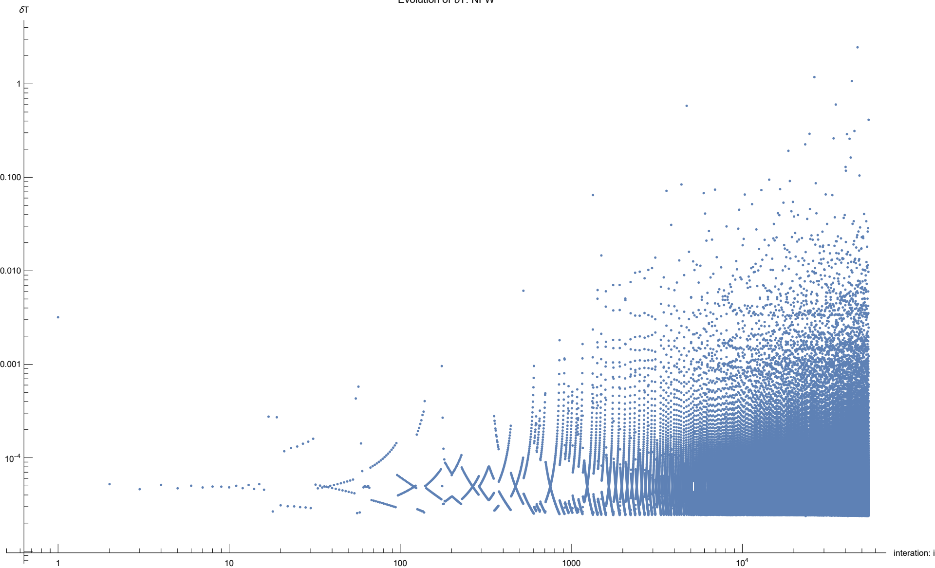
Evolution of \delta T : NFW
