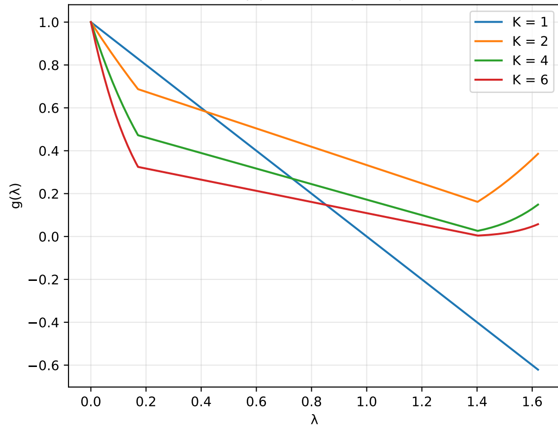
Коэффициенты фильтра
