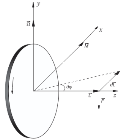
Рис. 1: Маховик
