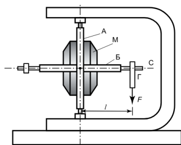
Рис. 2: Приложение 2. Схема маховика
