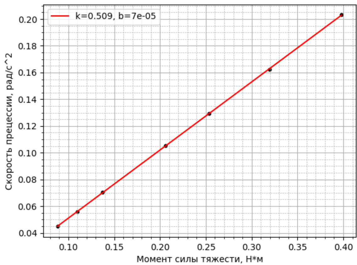
Рис. 3: Приложение 3. График зависимости угловой скорости прецессии от приложенного момента силы тяжести
