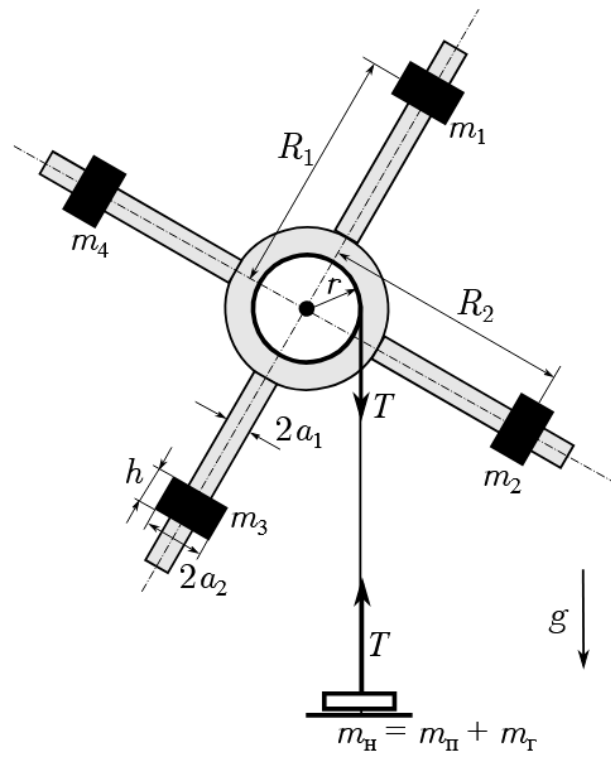
Рис. 1: Приложение 1: Маятник Обербека
