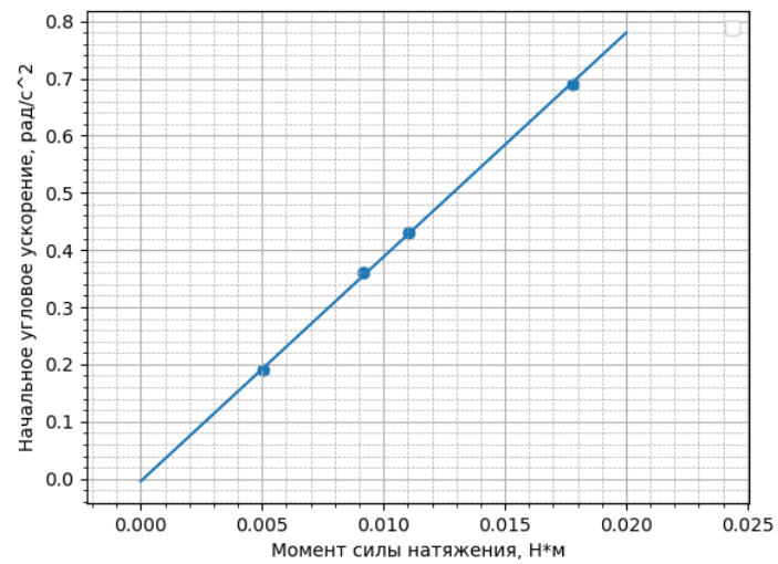
Рис. 2: Приложение 2: Зависимость углового ускорения от момента прикладываемой силы
