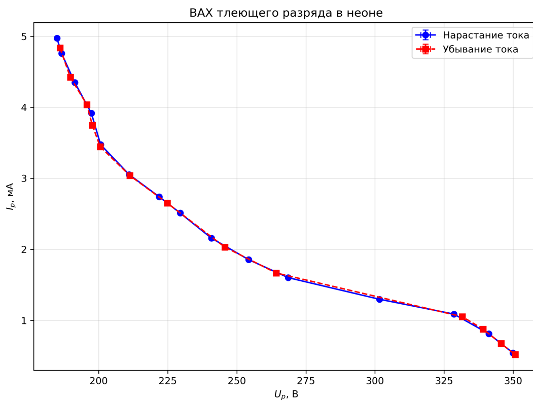
Приложение 2. ВАХ тлеющего разряда
