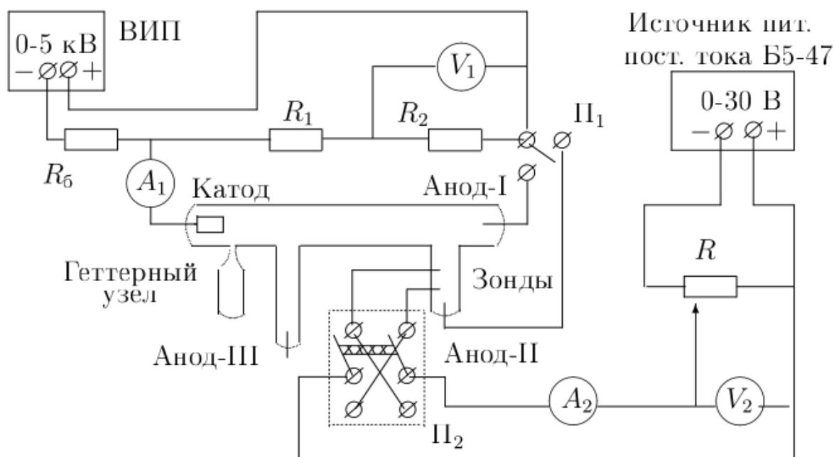
Рис. 1: Схема установки
