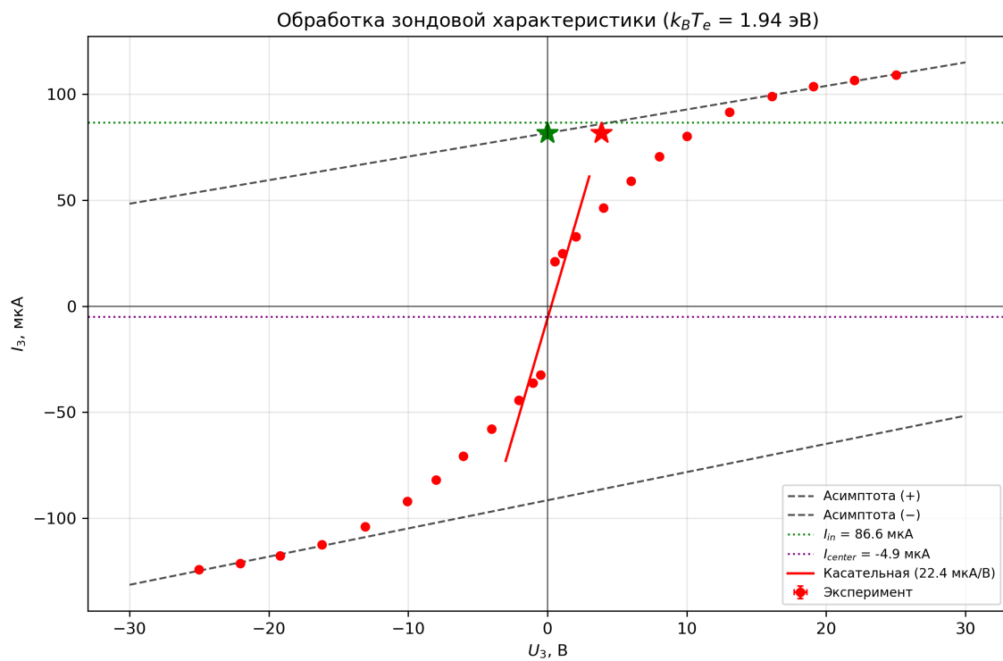
Рис. 3: Обработка зондовой характеристики для I_p = 4.99 мА: асимптоты, горизонталь I_{in} , касательная в нуле, точки 1 и 2
