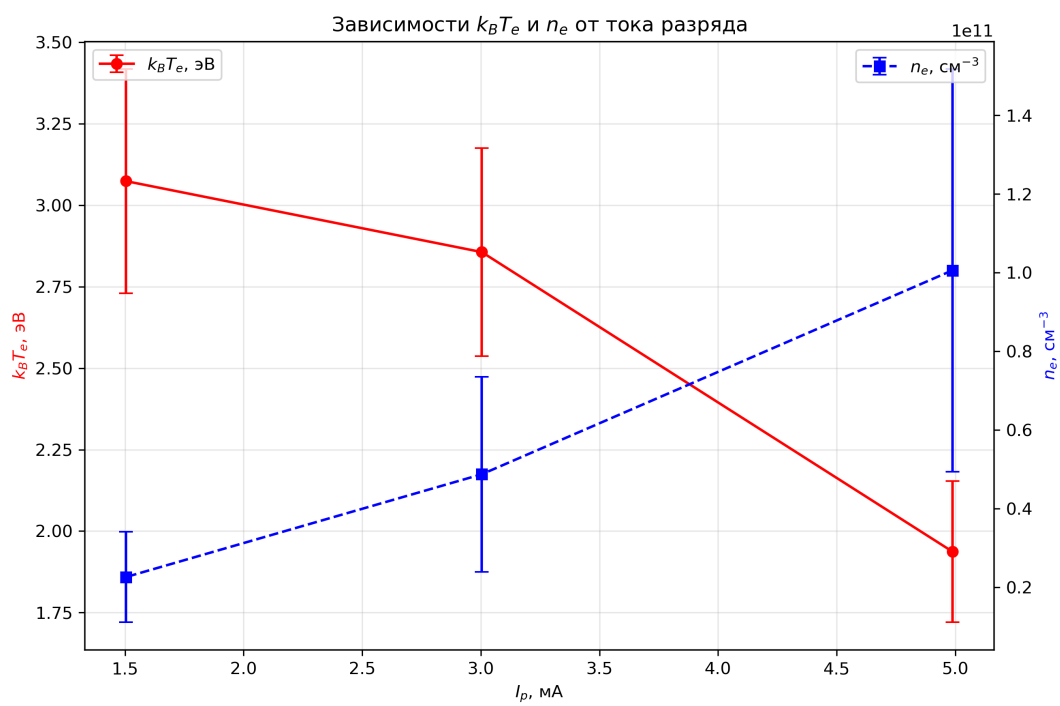
Приложение 5. Зависимости k_B T_e и n_e от тока разряда
