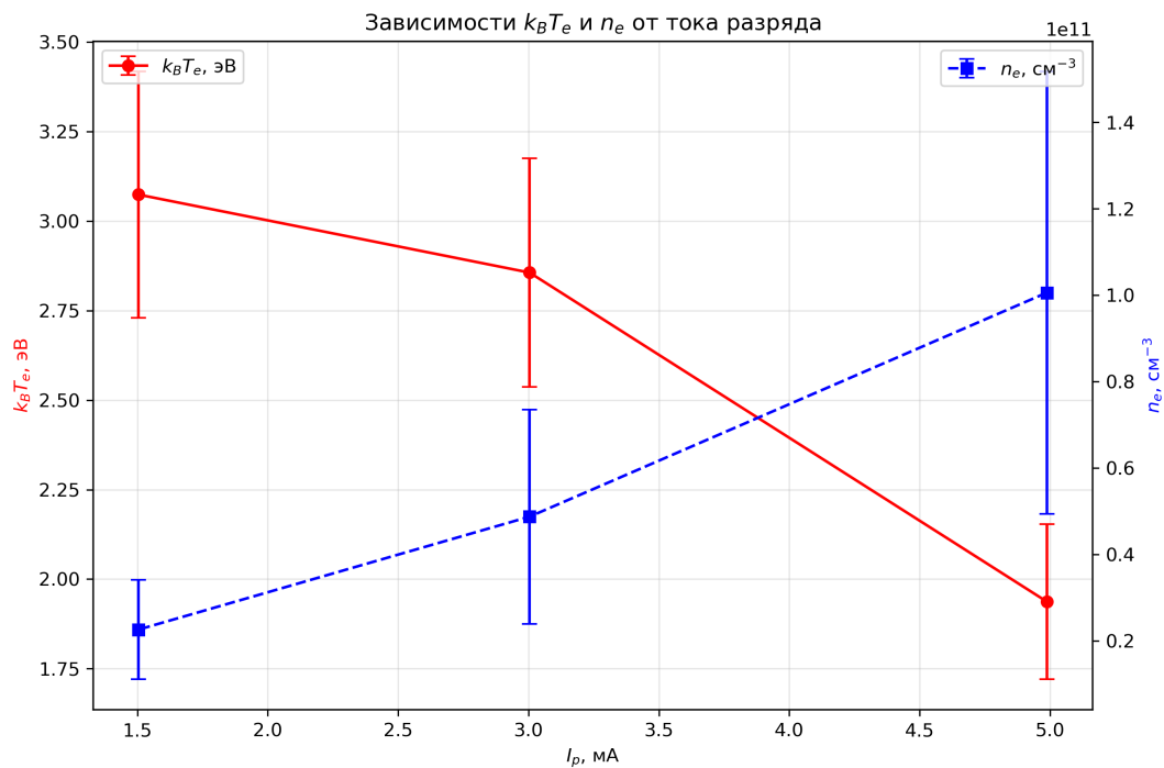
Рис. 5: Зависимости k_B T_e и n_e от тока разряда
