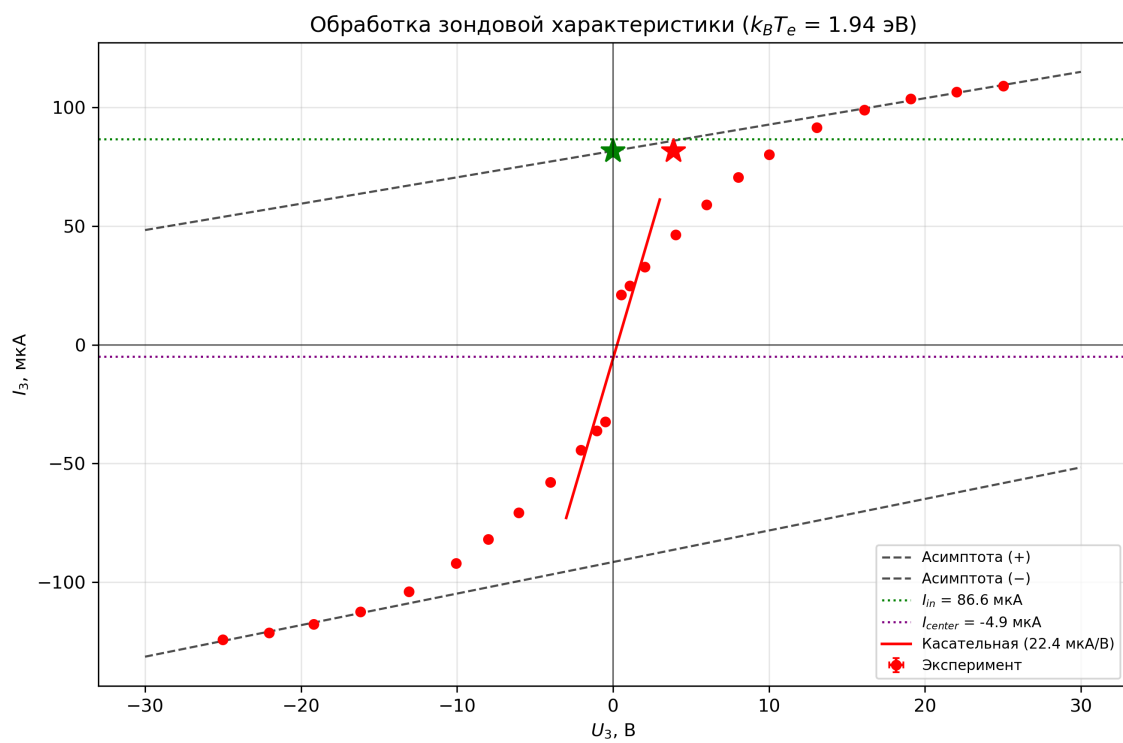
Приложение 4. Обработка зондовой характеристики
