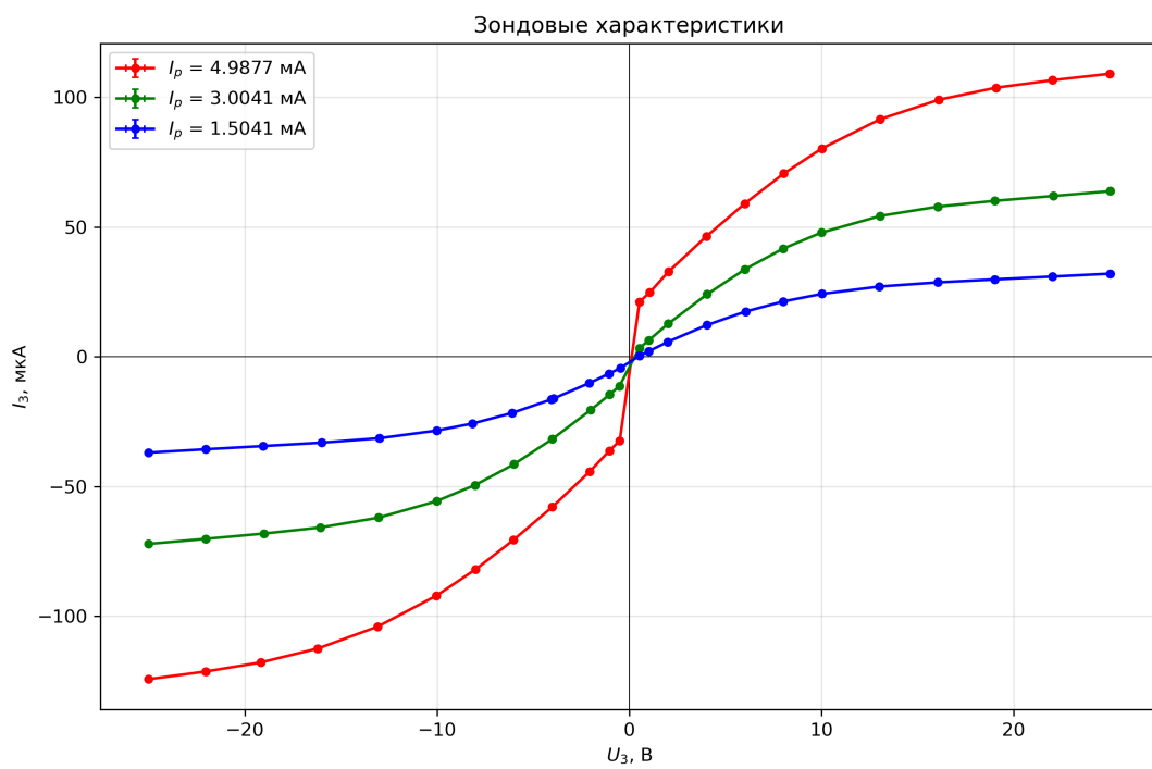
Рис. 4: Семейство зондовых характеристик
