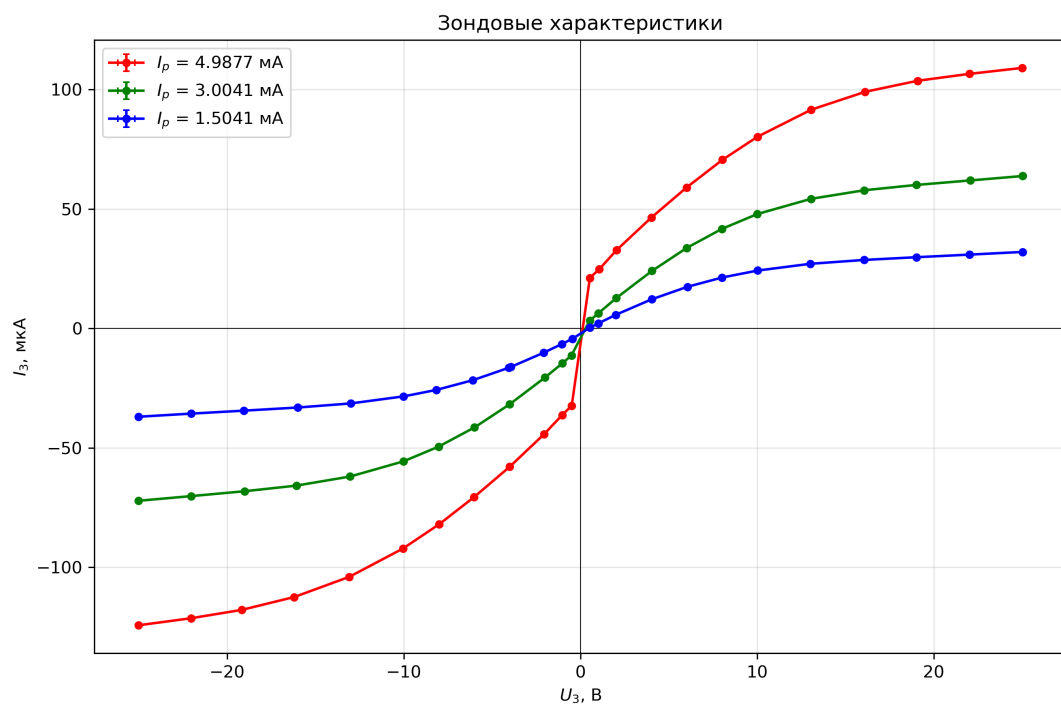
Приложение 3. Семейство зондовых характеристик
