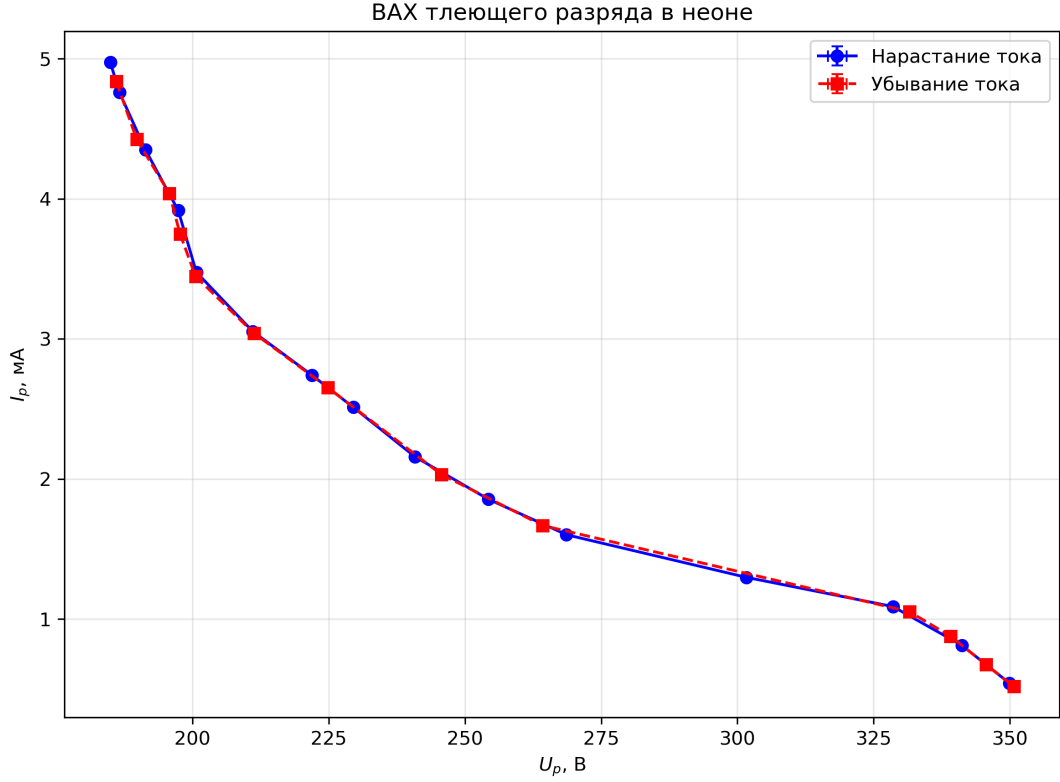
Рис. 2: Вольт-амперная характеристика тлеющего разряда в неоне
