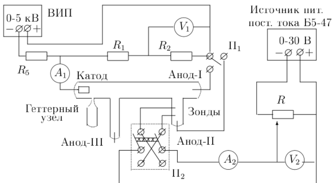
Приложение 1. Схема установки
