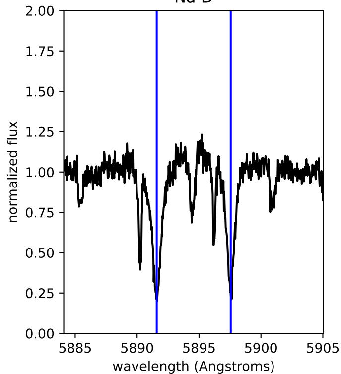
Na D
