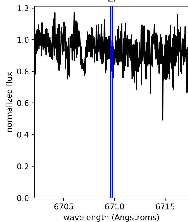
Li
