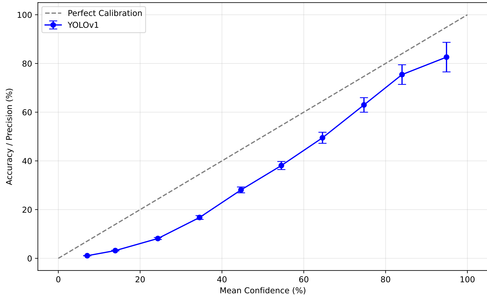
YOLOv1 Calibration
