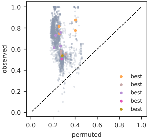
lobo3_f1_macro
