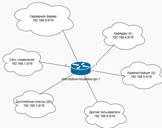
Рис. 5: Схема маршрутизации сети (Layer 3)
