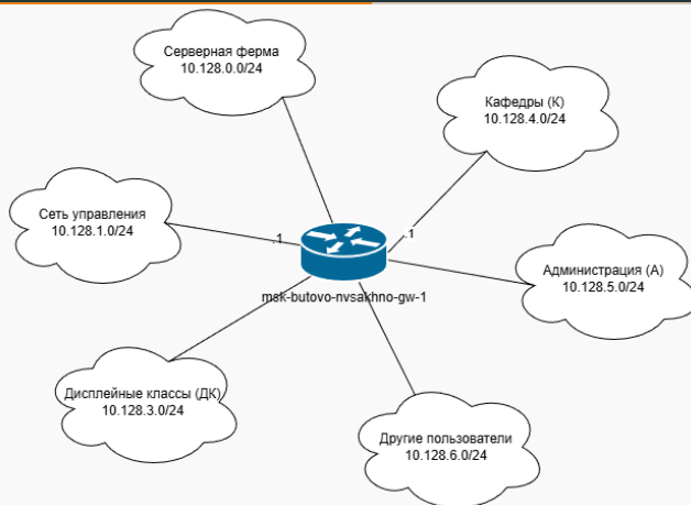
Рис. 3: Схема маршрутизации сети (Layer 3)
