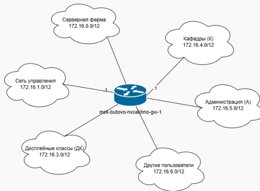
Рис. 4: Схема маршрутизации сети (Layer 3)
