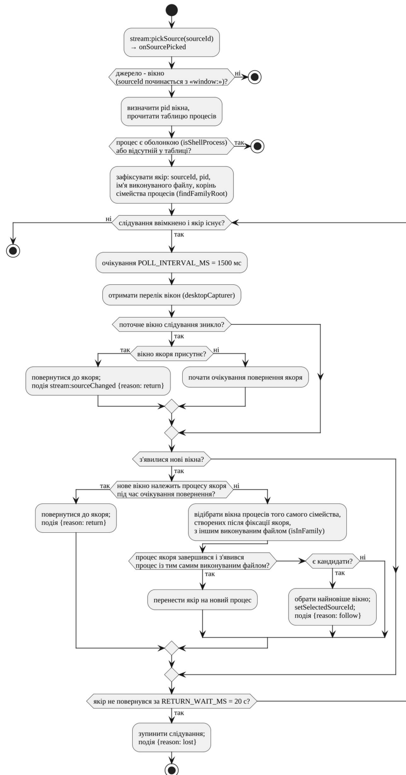
Рисунок 3.6 – Діаграма діяльності режиму слідкування за застосунком
