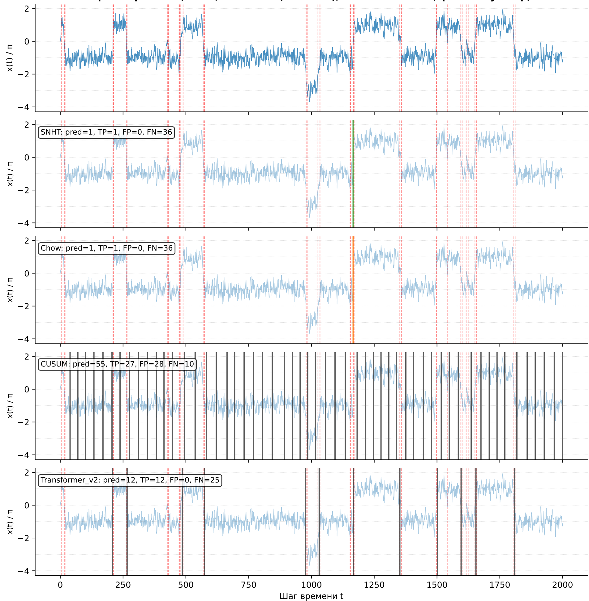
Траектория SDE (D=1.0, white noise, seed=42), истинные CP: 37 (красный пунктир)
