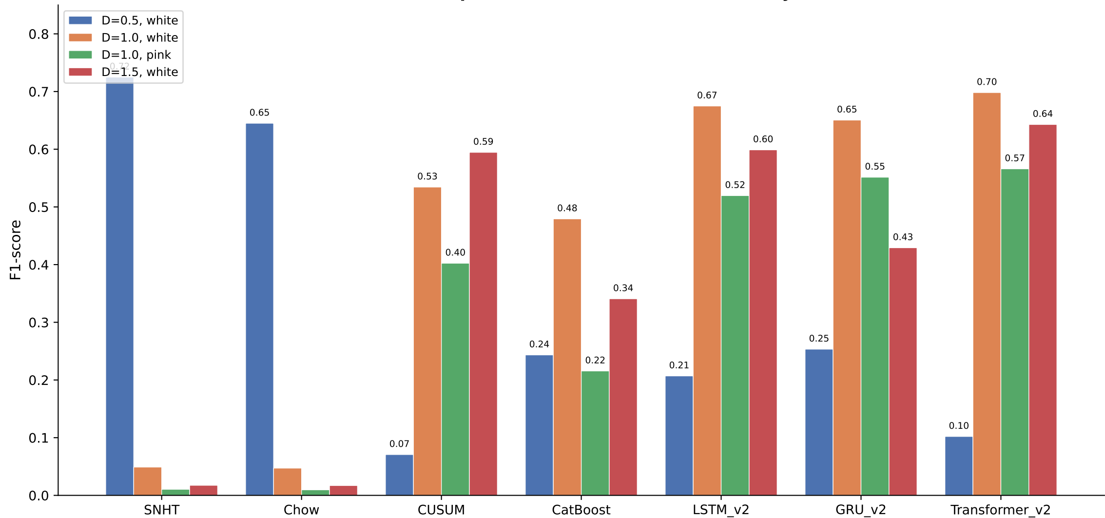
F1 по сценариям: зависимость от D и типа шума
