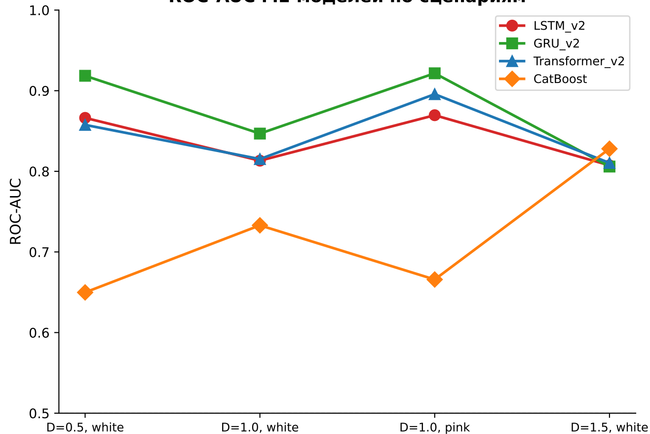
ROC-AUC ML-моделей по сценариям
