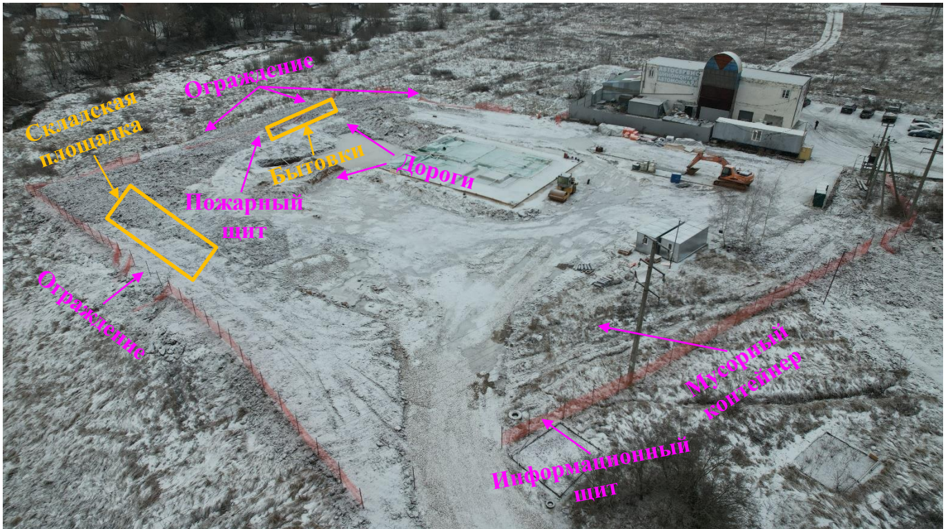
Фото 4 (Места устройства временных дорог, временных ограждений, мобильных зданий и сооружений, складских площадок, бункера для сбора мусора, информационного щита, стенда пожарной защиты согласно ПОС)
