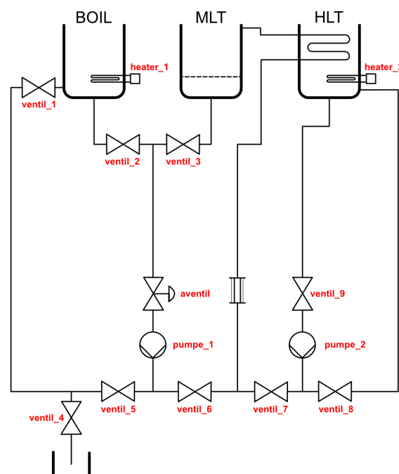
Abbildung 4: Nummerierung der Aktoren/Sensoren [3]
