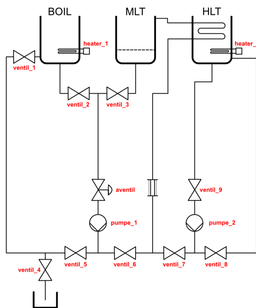
Abbildung 3: Nummerierung der Aktoren/Sensoren [2]
