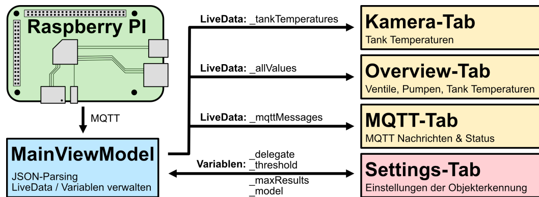
Abbildung 2: Überblick des Datenflusses der App
