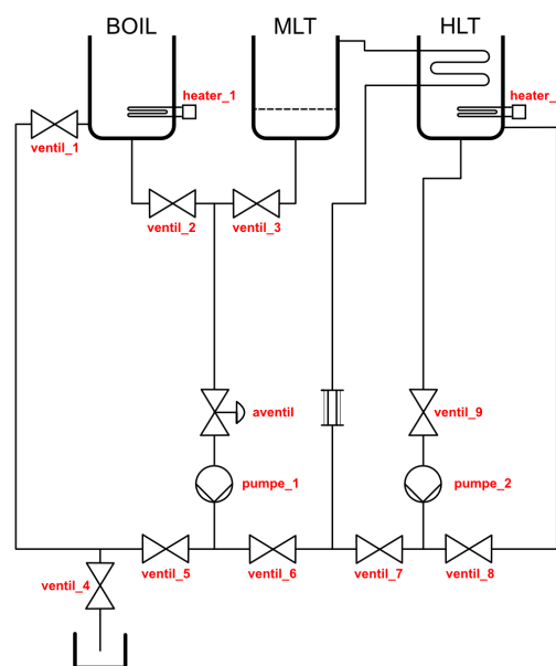
Abbildung 4: Nummerierung der Aktoren/Sensoren [3]
