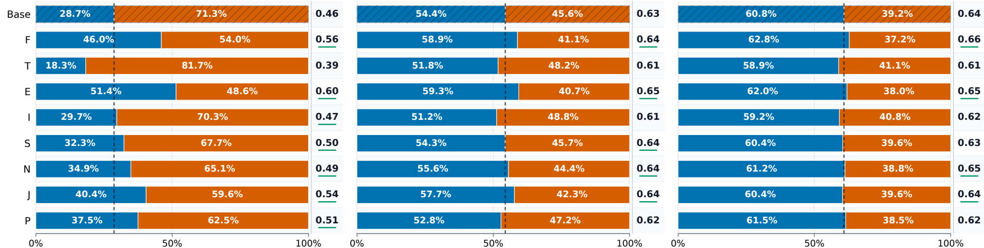
Llama-3.2-3B
