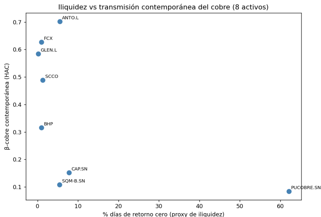
Figura 6. Il liquidez (porcentaje de días con retorno cero) frente a la elasticidad-cobre contemporánea de los ocho activos. Pucobre es el punto extremo de baja transmisión y alta il liquidez.
