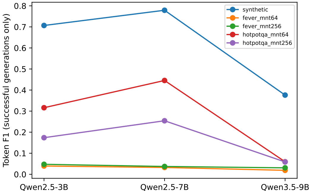
Token F1 vs. generator scale
