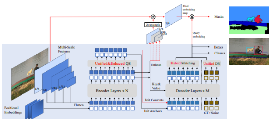
Σχήμα 4.1.1: Αρχιτεκτονική μοντέλου Mask DINO
