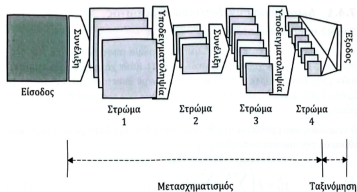
Σχήμα 2.4.1: Η αρχιτεκτονική ενός τυπικού συνελικτικού νευρωνικού δικτύου
