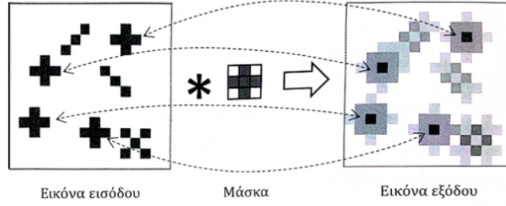
Σχήμα 2.4.3: Εξαγωγή χαρακτηριστικών
