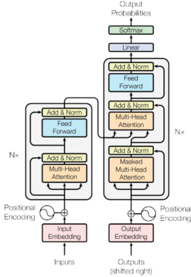
Σχήμα 2.5.1: Αρχιτεκτονική μετασχηματιστή
