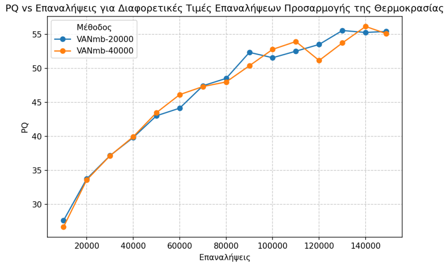
Σχήμα 6.5.1: Σύγκριση πανοπτικής ποιότητας για διαφορετικές τιμές των συνολικών επαναλήψεων προσαρμογής της θερμοκρασίας. VAN-20000: Πλήθος επαναλήψεων ίσο με 20000. VAN-40000: Πλήθος επαναλήψεων ίσο με 40000.
