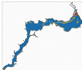
(h) S1 06-21 2077 km 2 dark
