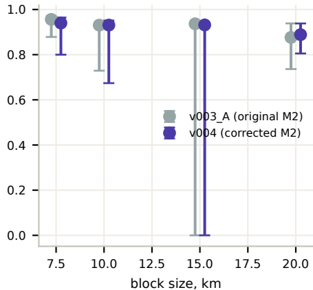
global F1 (weak labels)
