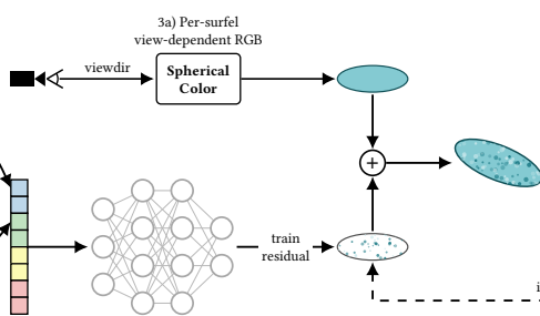
3b) view-independent MLP
