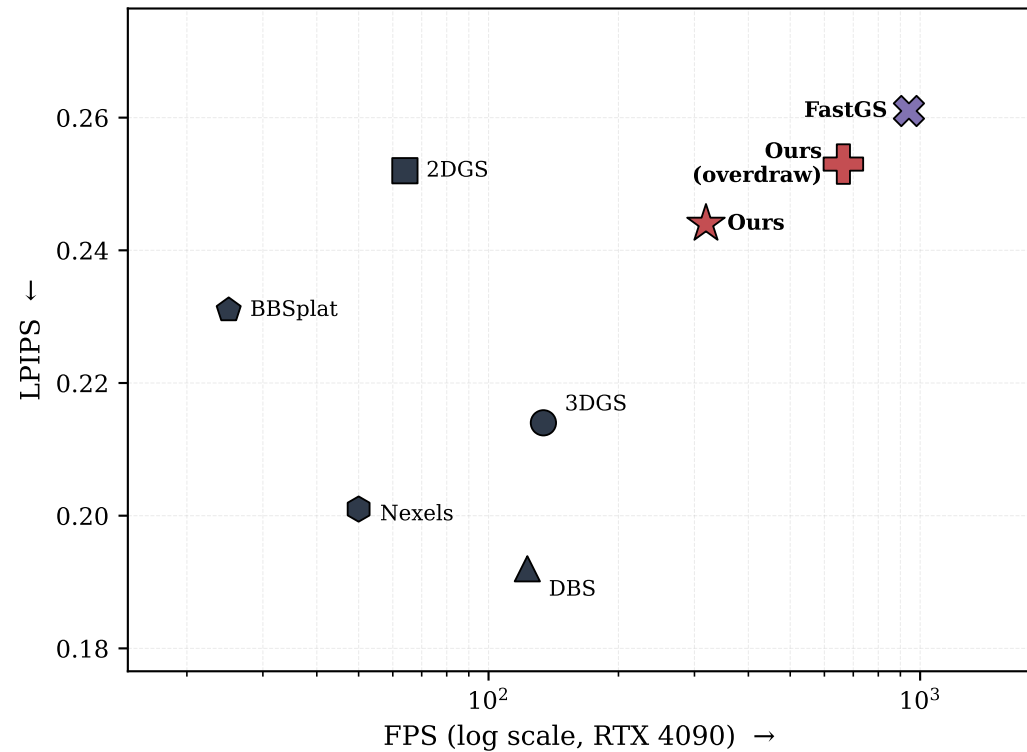
Mip-NeRF 360
