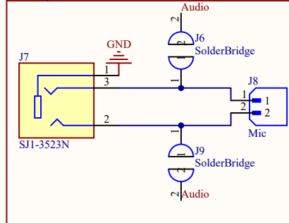
Audio input
