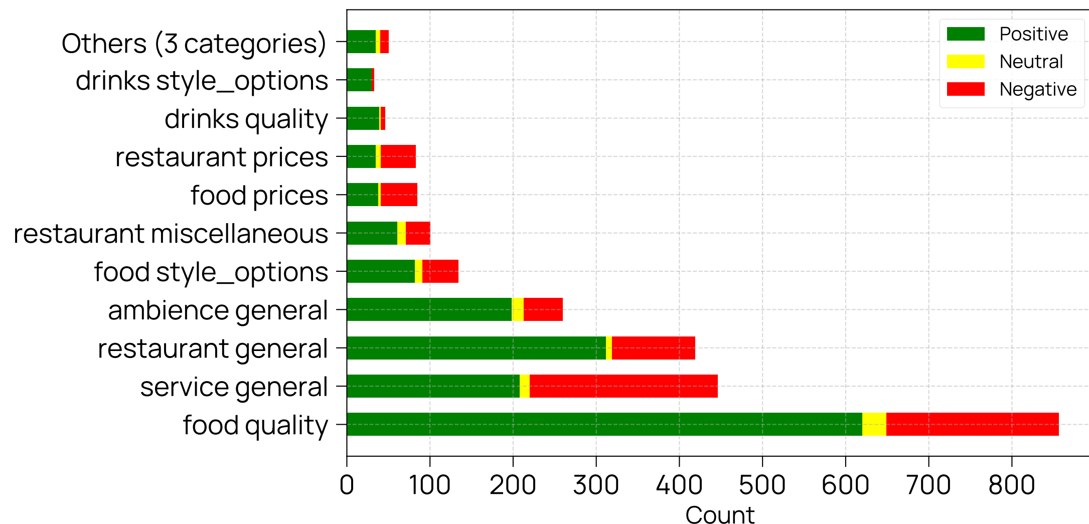
Rest16 - TASD
