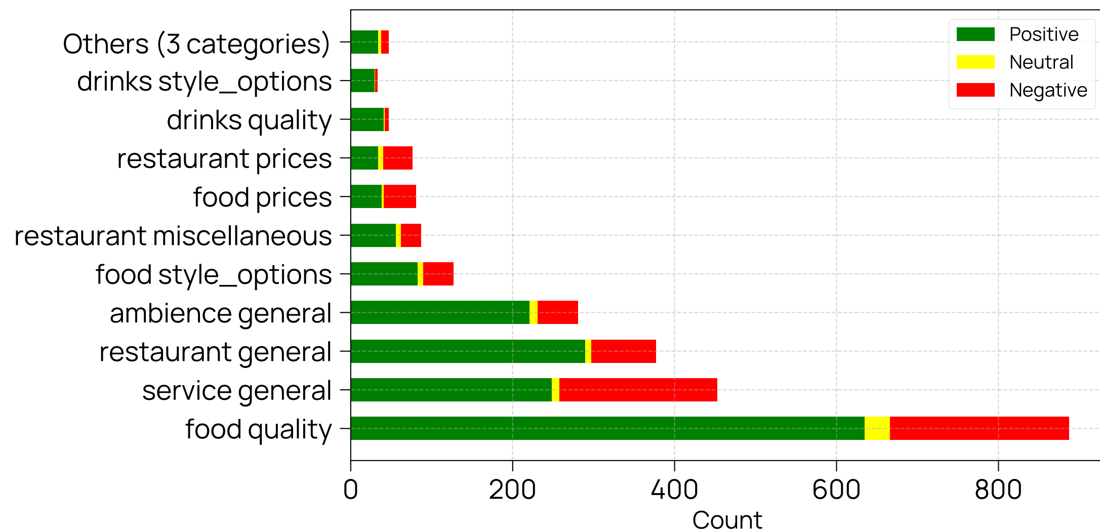
Rest16 - ASQP
