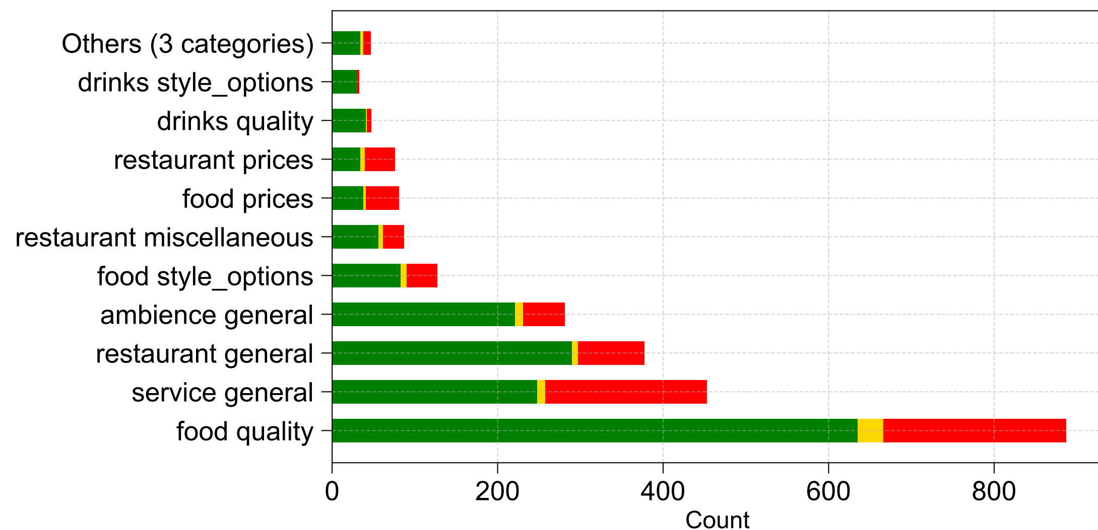
Rest16 - ASQP
