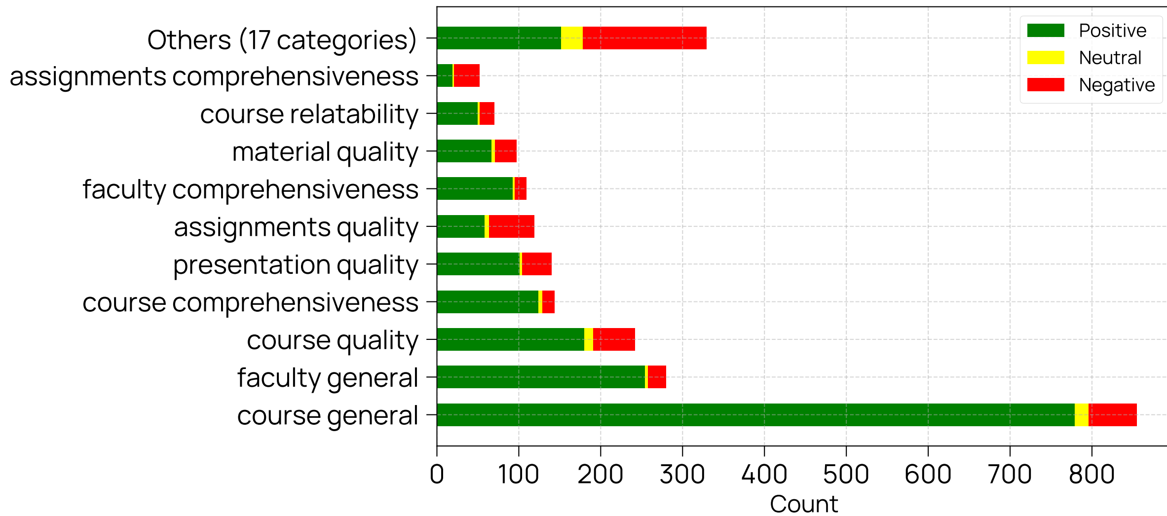
Coursera - TASD
