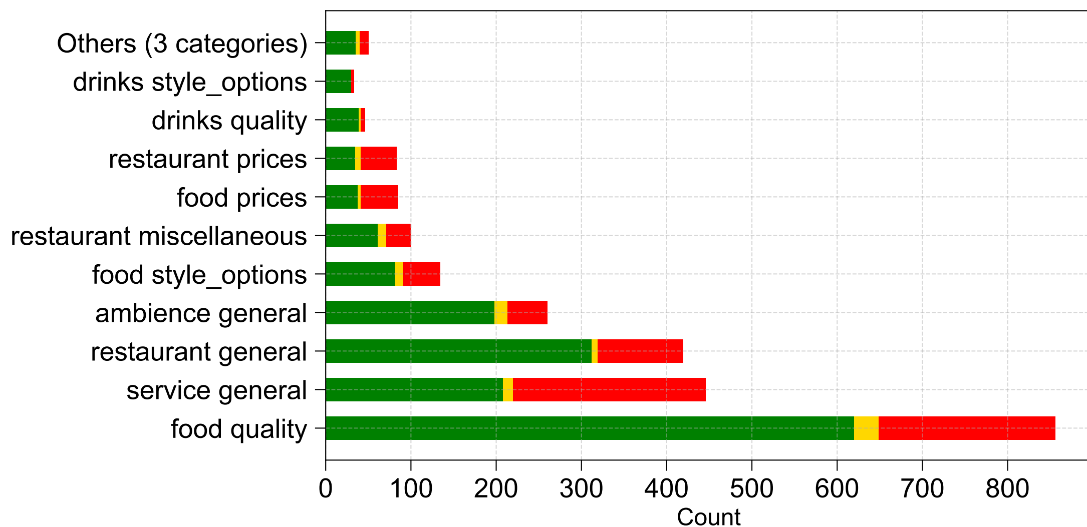
Rest16 - TASD
