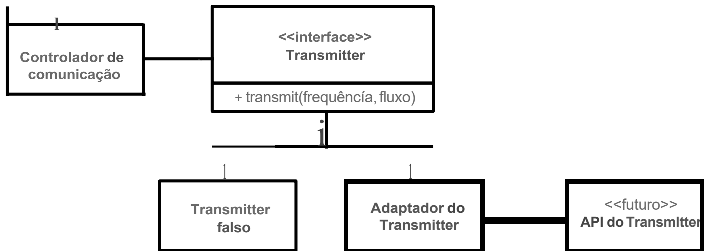
Figura 8.2: Adivinhando deverá ser o transmitter
