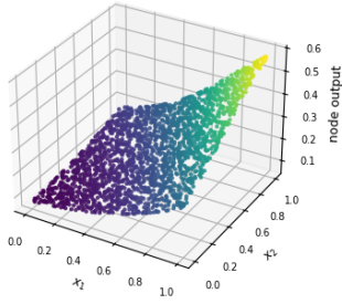
Bivariate regression dataset (2-D input) - FCNN 2-64-32-1 Hidden layer 2 node 4 - test data
