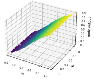
Bivariate regression dataset (2-D input) - FCNN 2-64-32-1 Hidden layer 1 node 6 - test data
