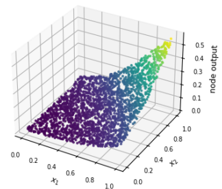
Bivariate regression dataset (2-D input) - FCNN 2-64-32-1 Hidden layer 2 node 6 - val data
