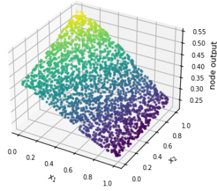
Bivariate regression dataset (2-D input) - FCNN 2-64-32-1 Hidden layer 2 node 5 - test data
