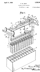
US-1579744-A · drawing
