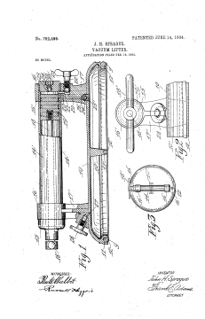
US-762499-A · drawing
