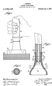
US-1178147-A · drawing
