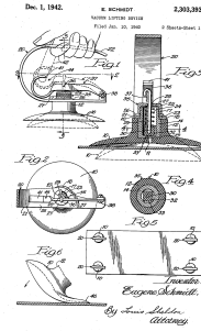
US-2303393-A · drawing
