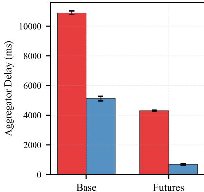
Monte Carlo
