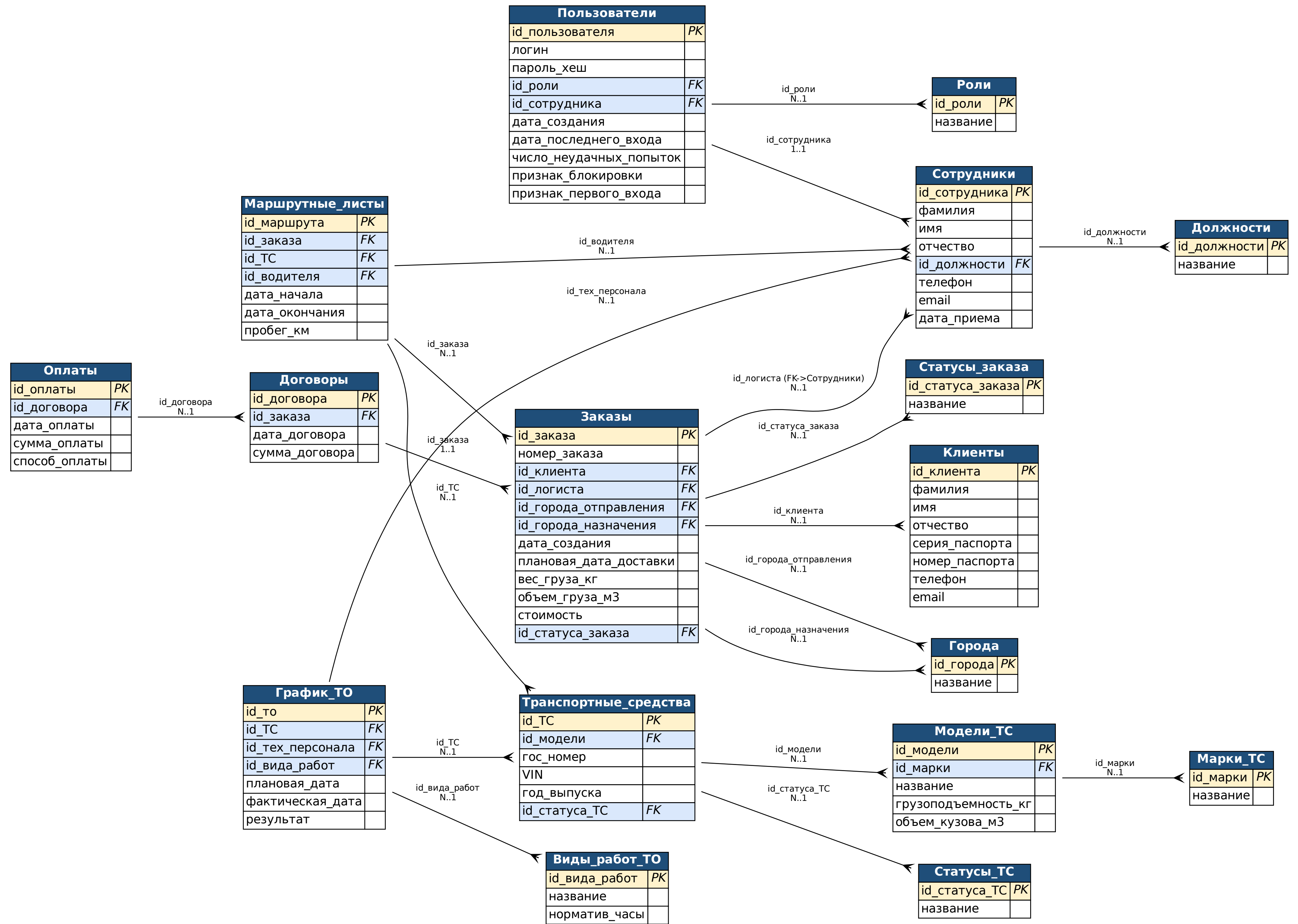
ER-диаграмма информационной системы транспортной компании (ЗНФ, ссылочная целостность через внешние ключи)
