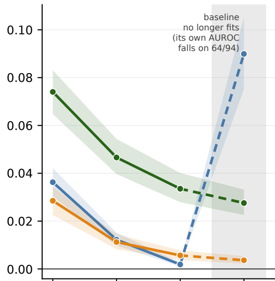
c bias-aware
