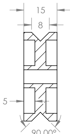
NUT
