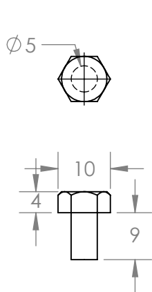
BOLT
