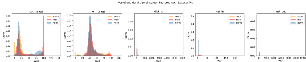
Abbildung 1: Verteilung der fünf universellen Features nach Datensatztyp (anom, mali, norm).
