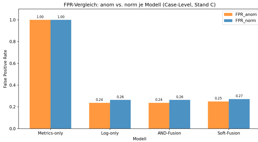
Abbildung 7: Vergleich von FPR_{anom} und FPR_{norm} zwischen Metrik-Baseline, Log-Komponente und den beiden Fusionsvarianten (Case-Ebene, n = 253 ).
