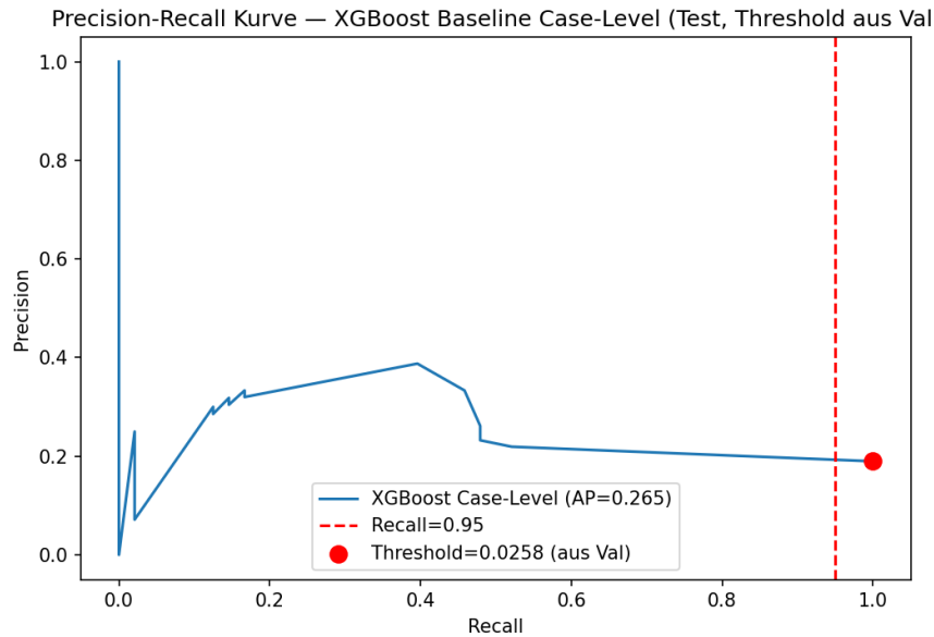
Abbildung 2: Precision-Recall-Kurve der Metrik-Baseline (AP = 0,2652, Case-Ebene). Der markierte Punkt entspricht dem Threshold 0,026 (aus Validierungsset) bei \text{Recall}_{\text{mali}} = 1,0000 .
