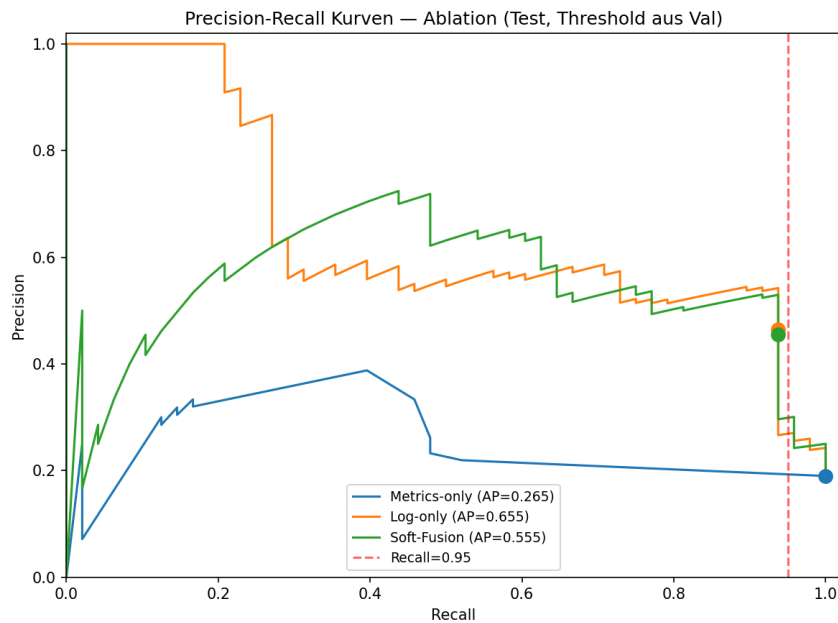
Abbildung 6: Precision-Recall-Kurven der Case-Level-Ablation. Die Metrik-only-Kurve basiert auf dem Case-Level-Score des XGBoost-Modells. Die Soft-Fusion-Kurve basiert auf dem Produkt-Score s = \hat{p}_{\text{metric}} \times \hat{p}_{\text{log}} . AND-Fusion hat keinen kontinuierlichen Score und erscheint nicht als Kurve. Alle AP-Werte beziehen sich auf dieselbe Granularität (Case-Ebene, n = 253 ).
