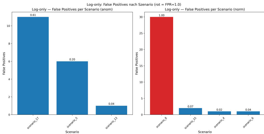
Abbildung 8: False Positives nach Szenario für Log-only, aufgeschlüsselt nach anom (links) und norm (rechts). Die Annotation zeigt die szenariospezifische FPR. Rote Balken markieren Szenarien mit FPR = 1,0 .
