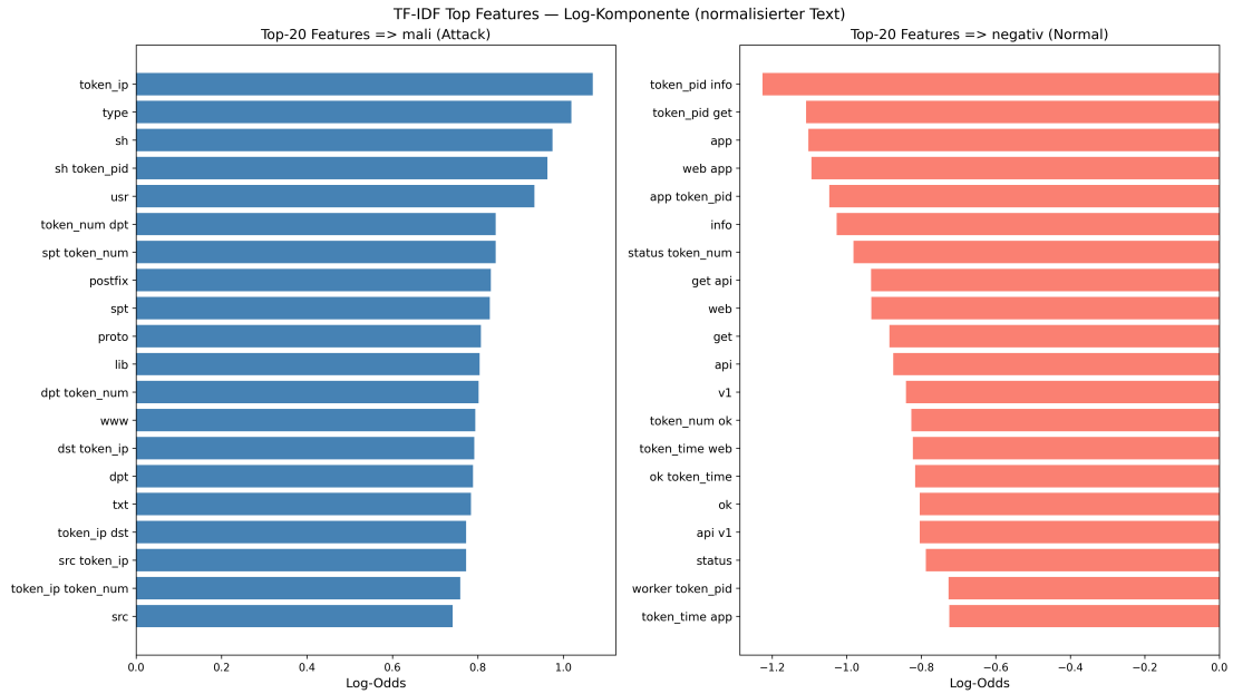
Abbildung 4: Top-20 TF-IDF-Terme nach Koeffizientengröße. Positiv gewichtete Terme sind stärker mit malignen Cases assoziiert. Negativ gewichtete Terme treten häufiger in benignen Cases auf.
