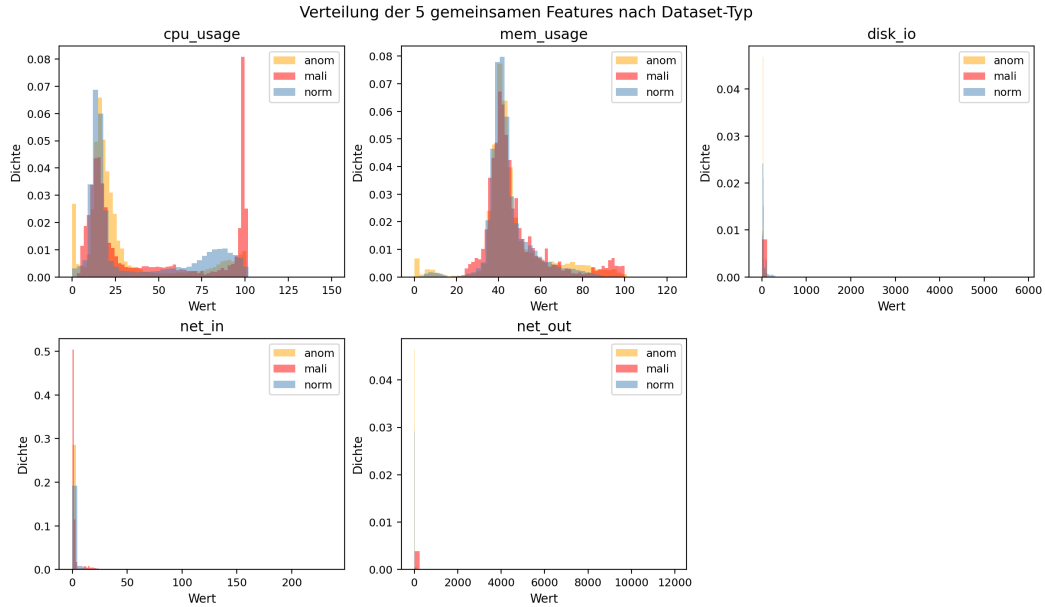
Abbildung 1: Verteilung der fünf universellen Features nach Datensatztyp (anom, mali, norm).
